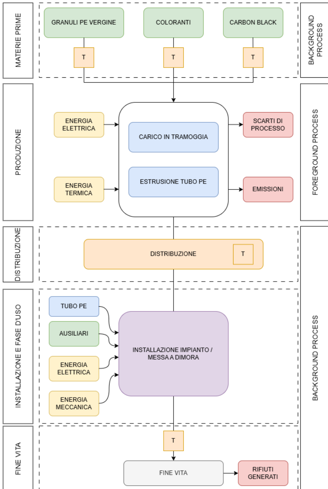
Figura 3 - Diagramma dei confini del sistema per le tubazioni oggetto di studio
